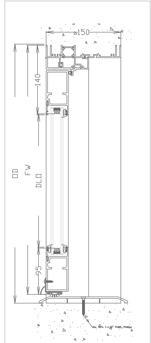
A-A
